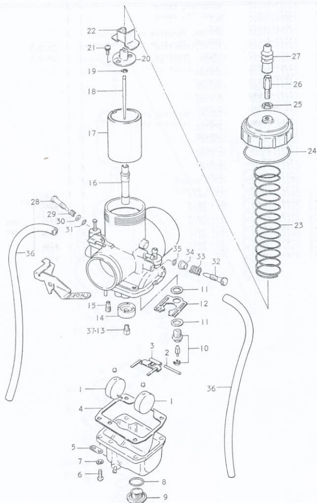
FIG.6 CARBURETOR (PE250N)
