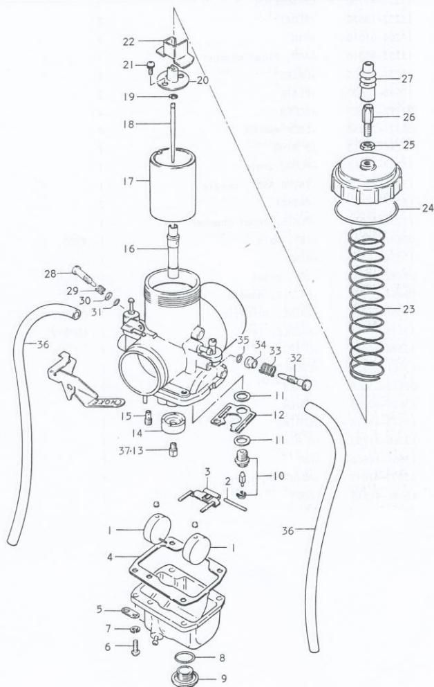
FIG.6 CARBURETOR (PE250N)
