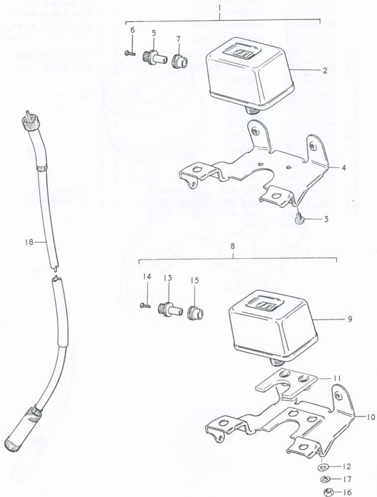
FIG.18 TRIP METER
