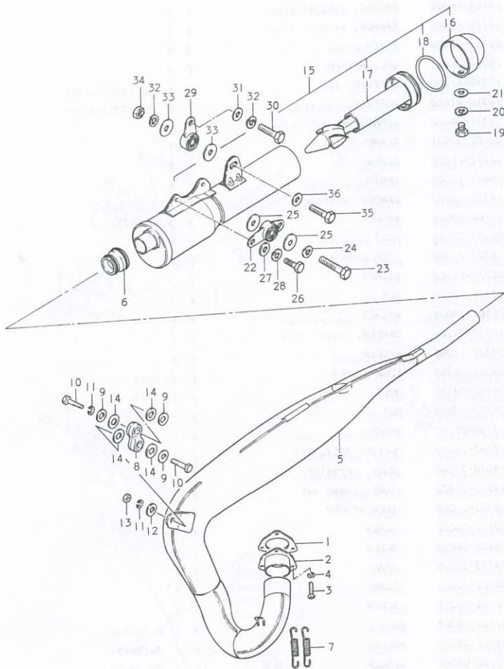
FIG.9 MUFFLER (PE250N)
