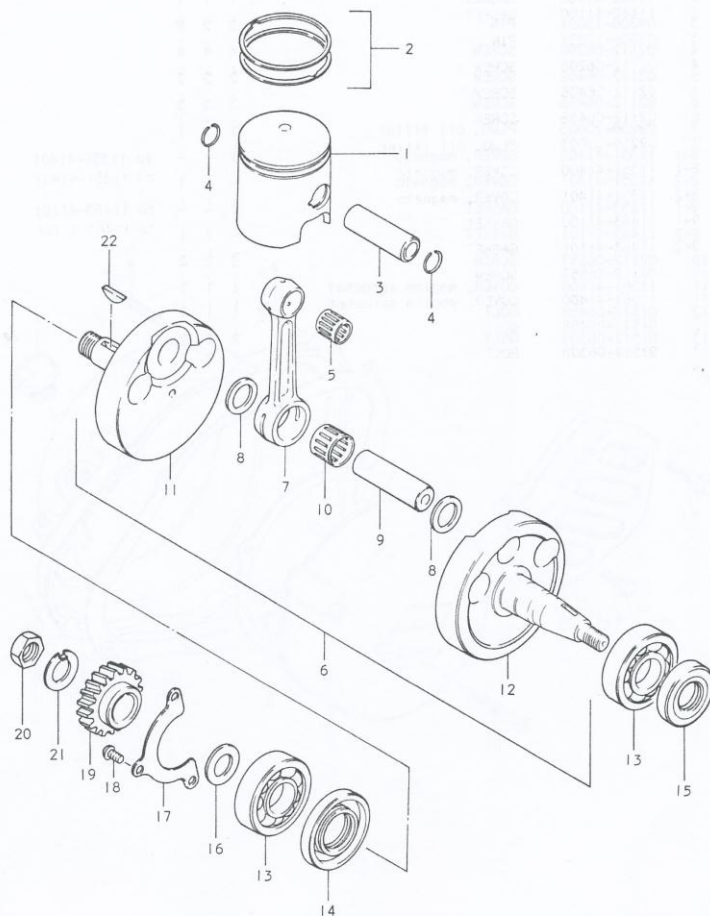
FIG. 4 CRANKSHAFT
